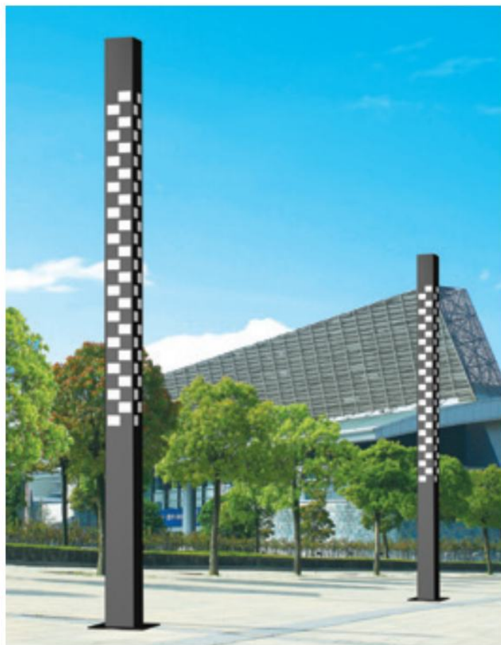
型号: LDJG-17504 型 高度:3-8m 光源: LED/ 节能灯
